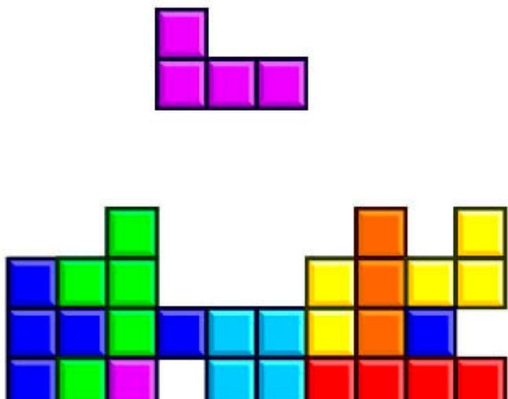
Tetris
